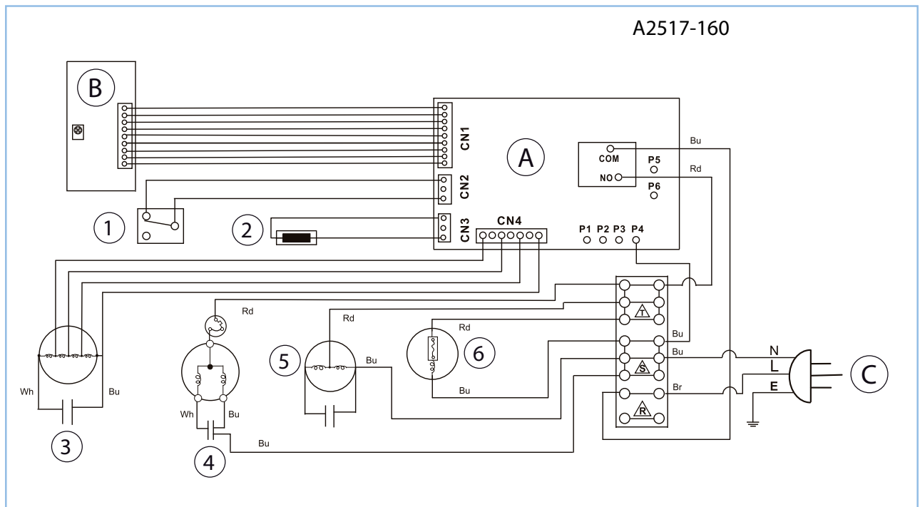
Abb. 1 : elektrisches Schaltschema
