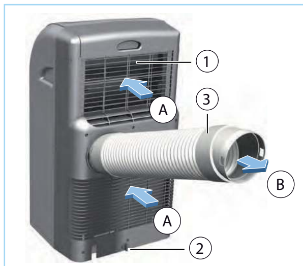
Abb. 2: Rückansicht
